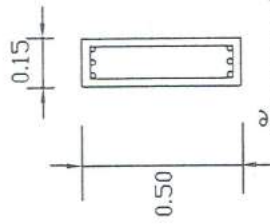
ตัดเสา C
